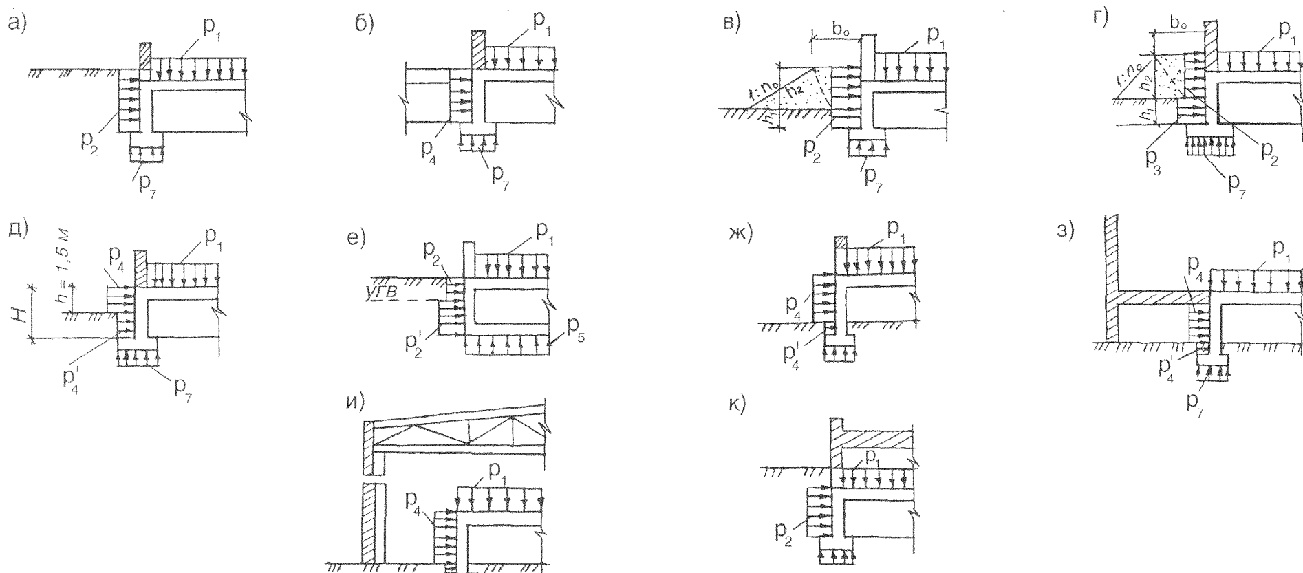
Рисунок 1 – Схеми прикладання динамічних навантажень на конструкції
